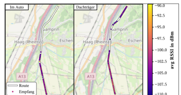
Vergleich der Senderposition Eigene Darstellung
