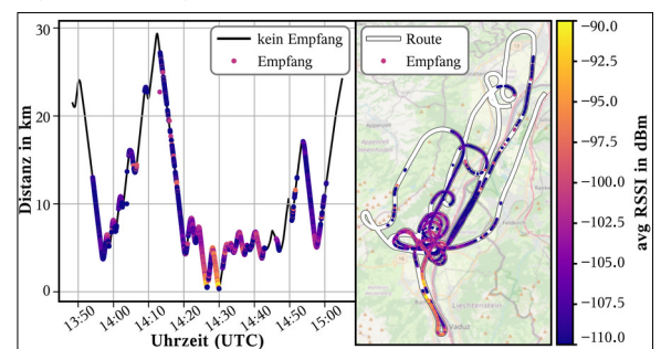
Auswertung des Flugtests Eigene Darstellung
